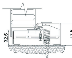
C-IK terskel
