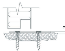
20 mm anslag
